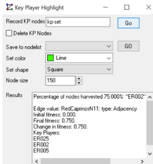
Figura 102. Resultado del procedimiento KPP-Pos, opción “Harvest”, con tres nodos y una distancia de 1, dos nodos (ER010 y ER018) se configuraron como intocables o no requeridos.
