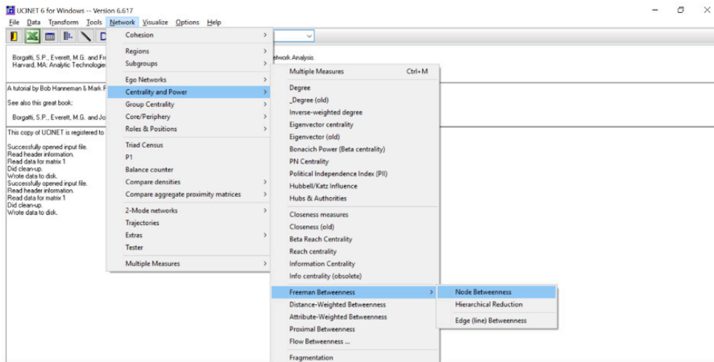
Figura 70. Menú para el cálculo de la centralidad de intermediación en UCINET.
