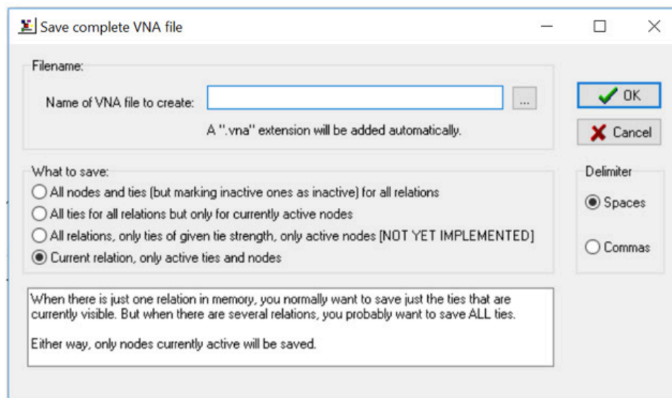
Figura 84. Creación del archivo VNA desde NetDraw.
