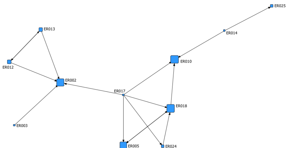
Figura 79. Gráfico de red con atributo Centralidad Beta de Bonacich por cada nodo, a mayor tamaño mayor valor de Centralidad Beta, y viceversa.
