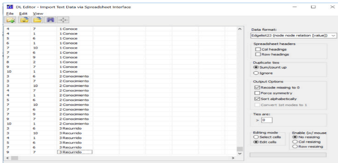
Figura 22. Datos de red de 10 nodos con formato Edgelist23 en el Editor DL de UCINET, para sistematizar tres tipos de relaciones entre los nodos de la red en un mismo archivo.
