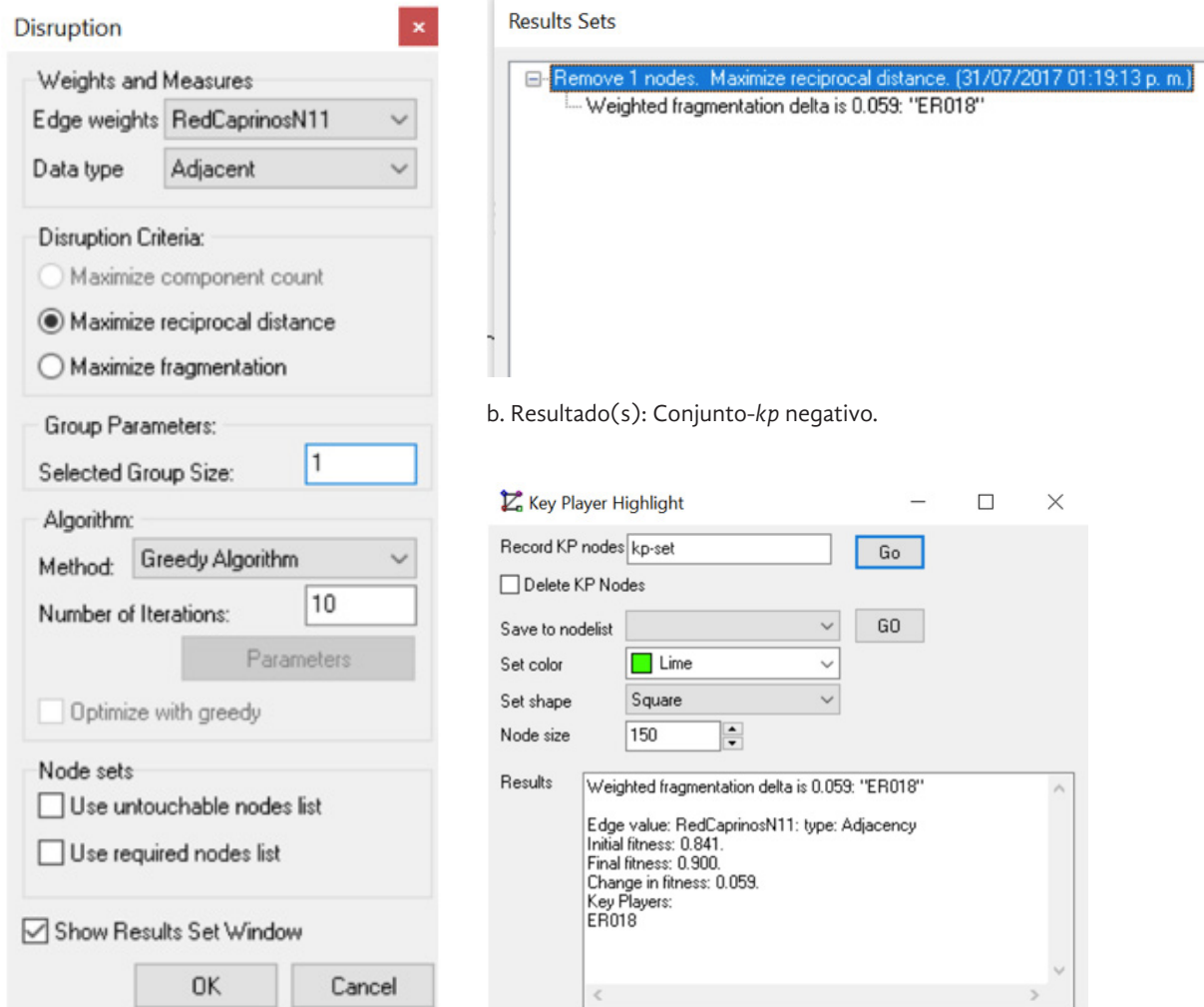
Figura 87. Configuración del procedimiento para obtener el KPP-Neg, en KeyPlayer 2.
