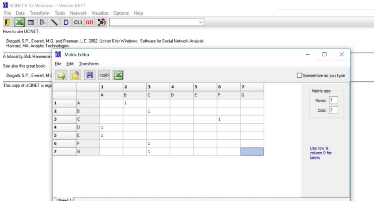
Figura 6. Datos del ejemplo copiados al Editor de matrices.
