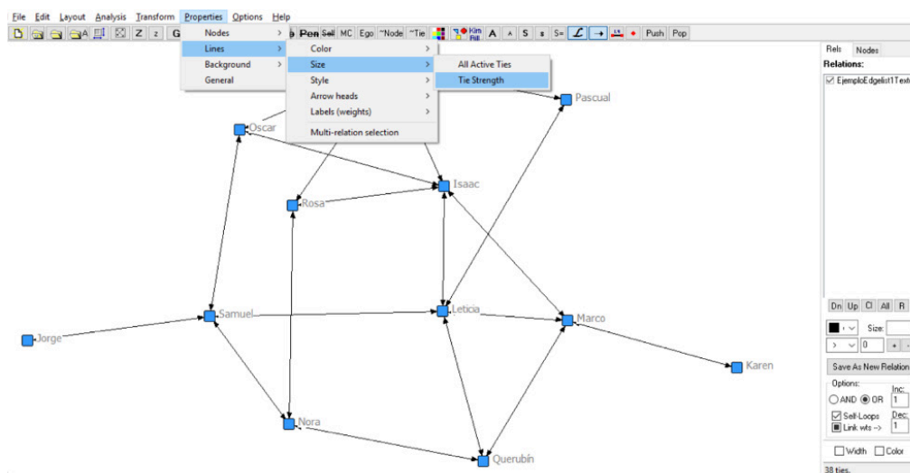
Figura 50. Menú para cambiar el grosor de las líneas entre los nodos, según intensidad del vínculo.
