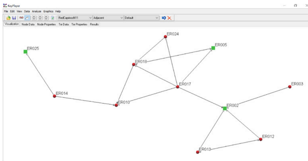
Figura 103. Conjunto- kp positivo de tres nodos (los nodos ER010 y ER018 fueron configurados como no requeridos, por ello no fueron seleccionados), procedimiento “Harvest”, en KeyPlayer 2.
