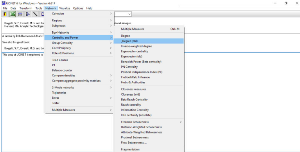
Figura 64. Menú para el cálculo de la centralidad de grado en UCINET.
