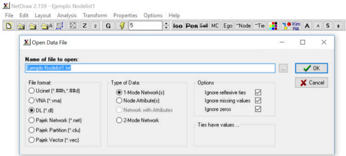
Figura 31. Apertura de archivo de texto DL con formato Nodelist1 con NetDraw.
