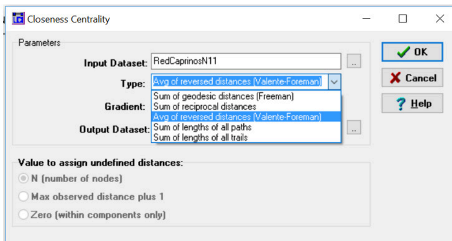
Figura 80. Configuración para el cálculo de la integración y radialidad en UCINET.
